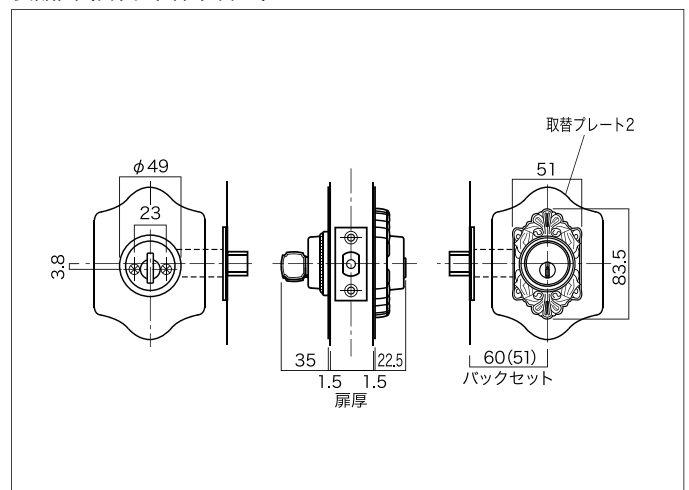
製品図 (古代 本締取替錠)
