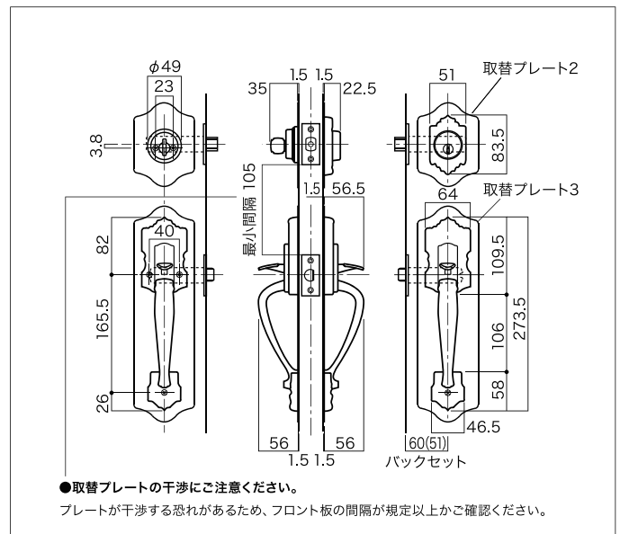
製品図 (古代 他社取替対応錠)
