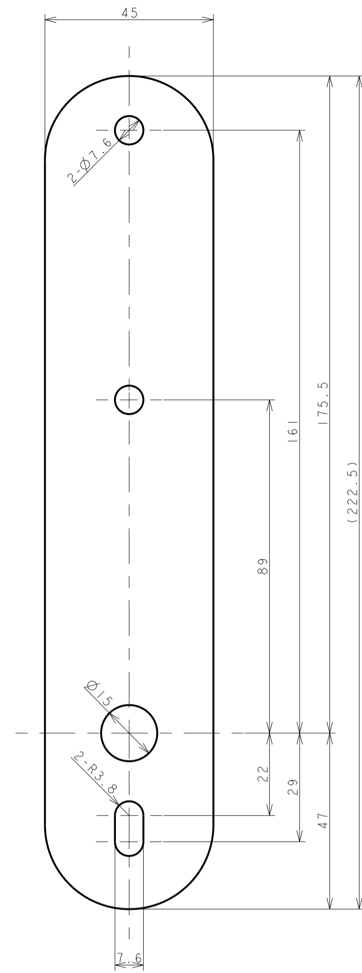
ロックベーススペーサー 厚み1.0mm/2.0mm/3.0mm
