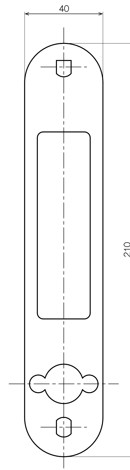
調整用スペーサー 厚み2mm
