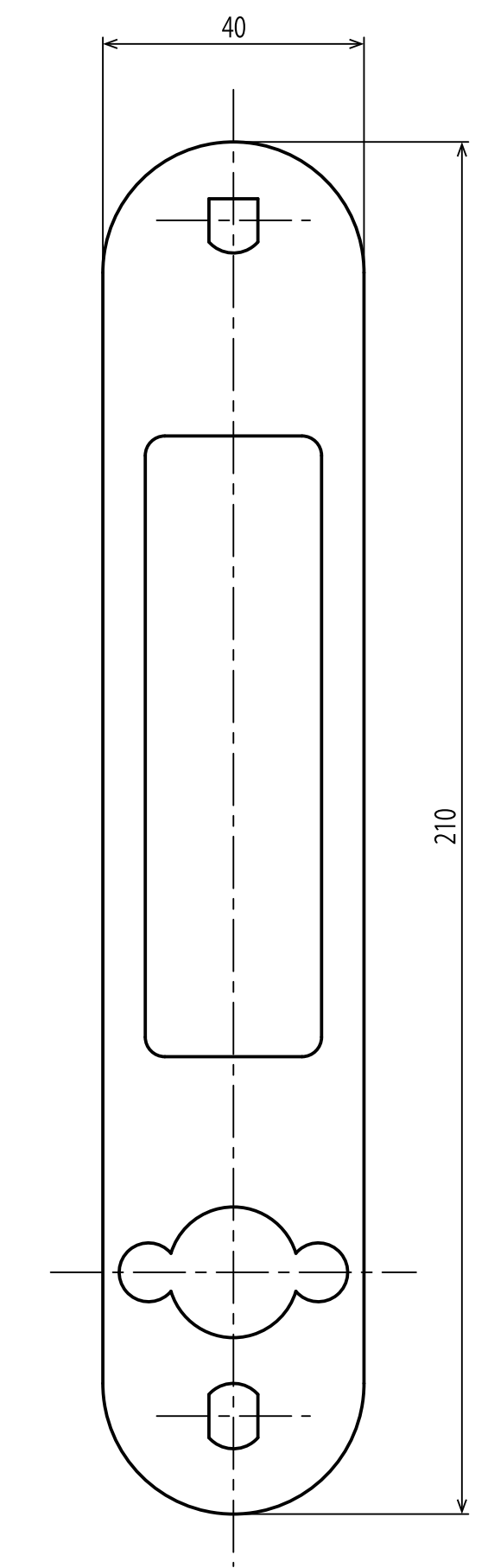
調整用スペーサー 厚み2mm
